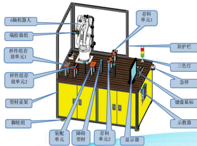
机器人示教平台 Robot teaching platform
